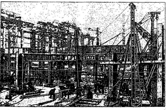
Aanleg van een groot krachtwerk te Rummelsburg te Berlijn, waarbij een groot aantal werklozen arbeid vinden.
